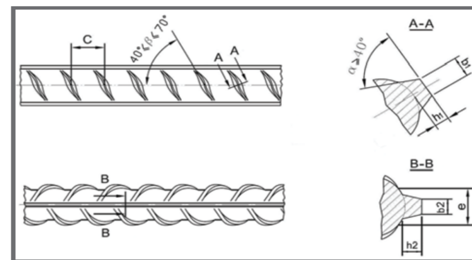
ویژگی ابعادی میلگرد A3
